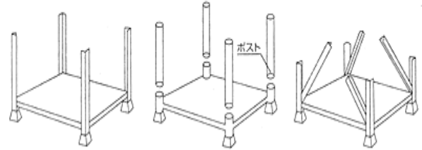
図14-a 固定式 ポストパレット 図14-b 取外し式 図14-c 折たたみ式
