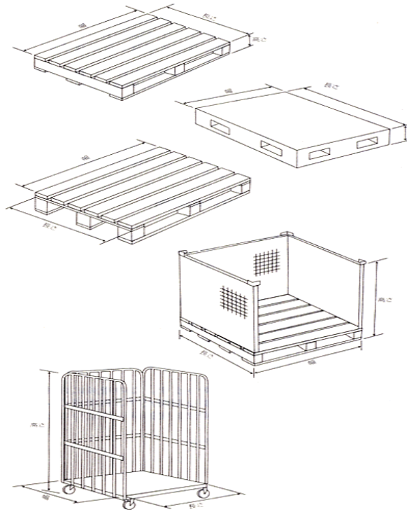
図51 パレットの長さ、幅、高さ
